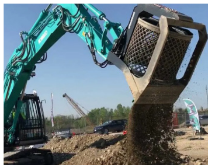
Sieblöffel
